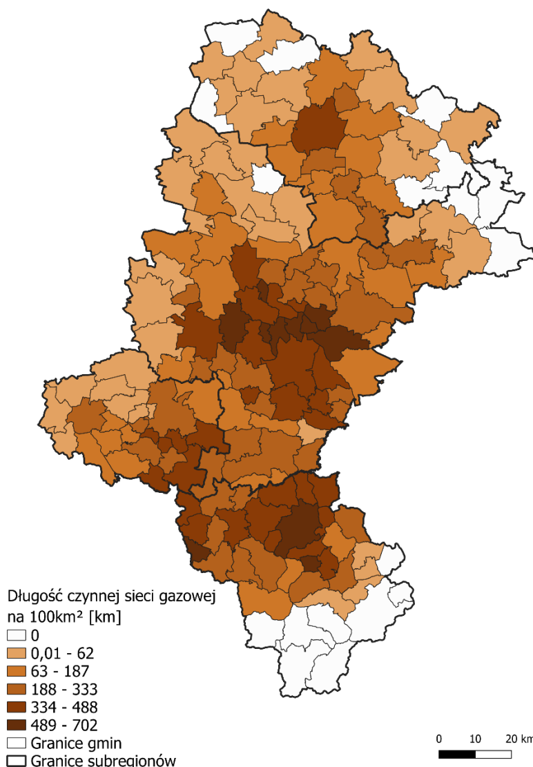
Mapa 4. Gęstość sieci gazowej województwa śląskiego w roku 2023
