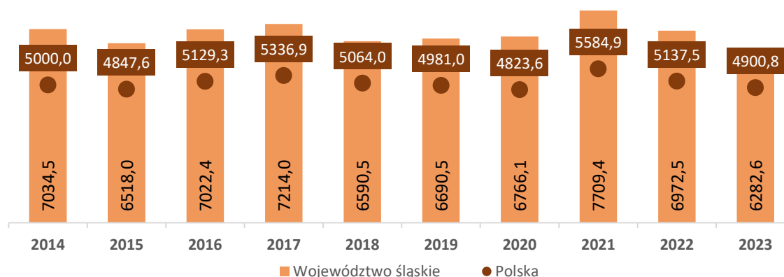
Wykres 3. Sprzedaż energii ciepłej w ciągu roku dla województwa śląskiego w latach 2014–2023
