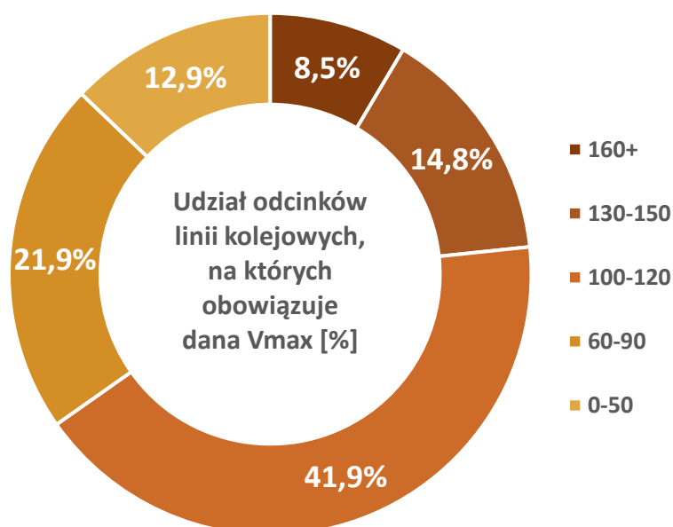
Wykres 10. Udział odcinków linii kolejowych, na których obowiązuje dana Vmax [%]
