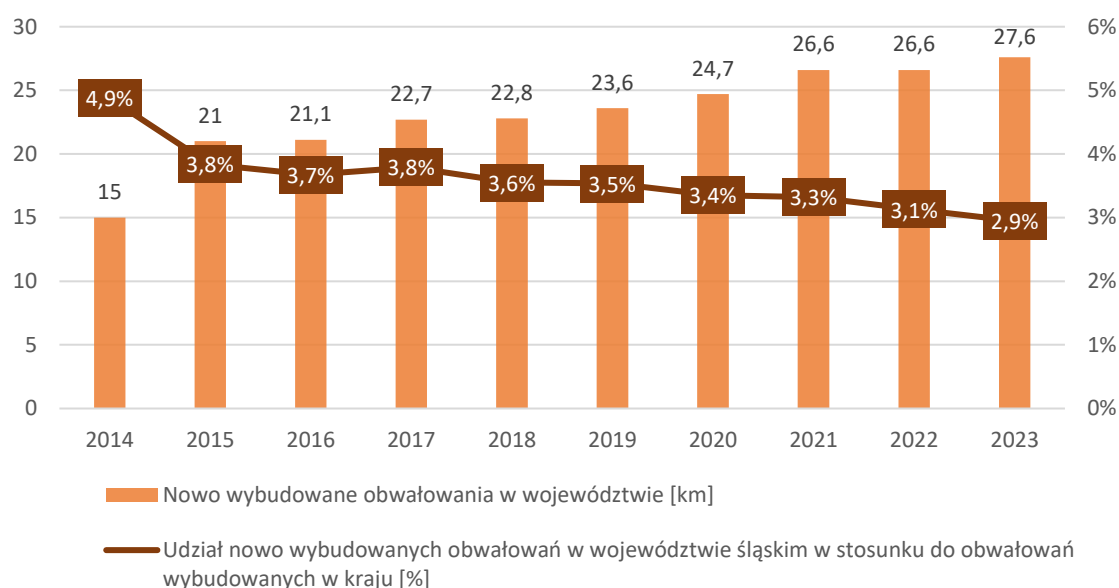
Wykres 15. Skumulowana długość nowo wybudowanych obwałowań przeciwpowodziowych [km] w województwie śląskim w latach 2014-2023
