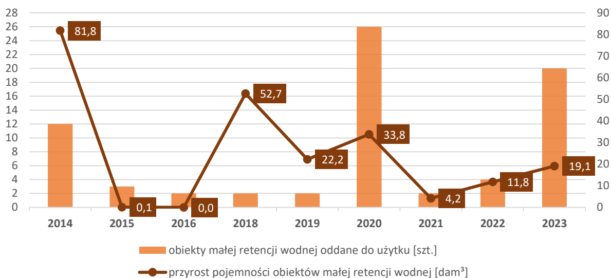
Wykres 14. Efekty rzeczowe inwestycji malej retencji wodnej w województwie śląskim w latach 2014-2023
