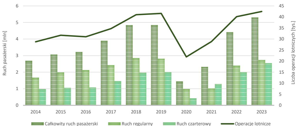
Wykres 30. Liczba pasażerów obsługiwanych przez MPL „Katowice” w Pyrzowicach i operacje lotnicze w latach 2014-2023.
