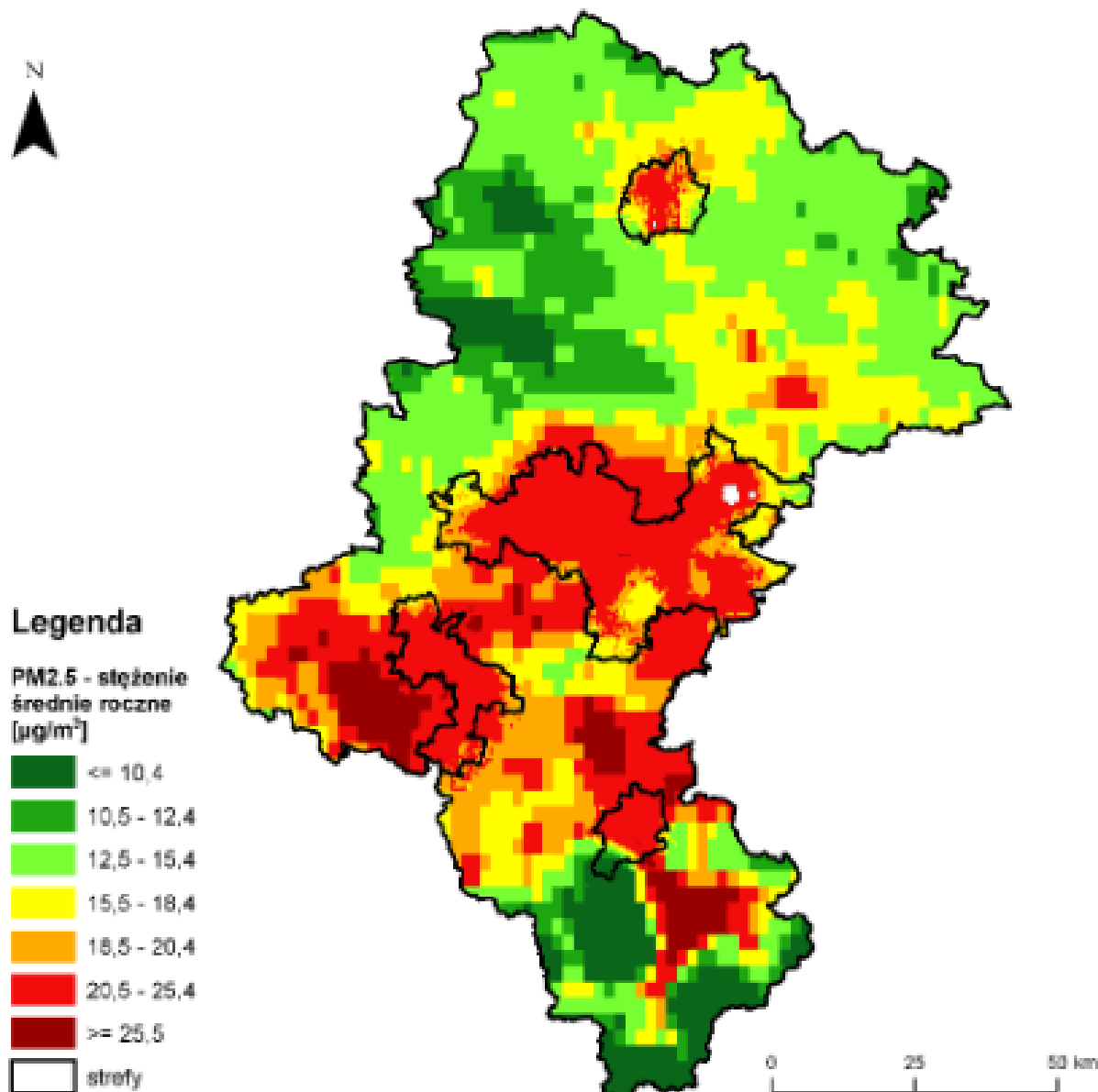
Mapa 24. Rozkład przestrzenny średniorocznego stężenia pyłu PM 2,5 na obszarze województwa śląskiego w 2021 roku.
