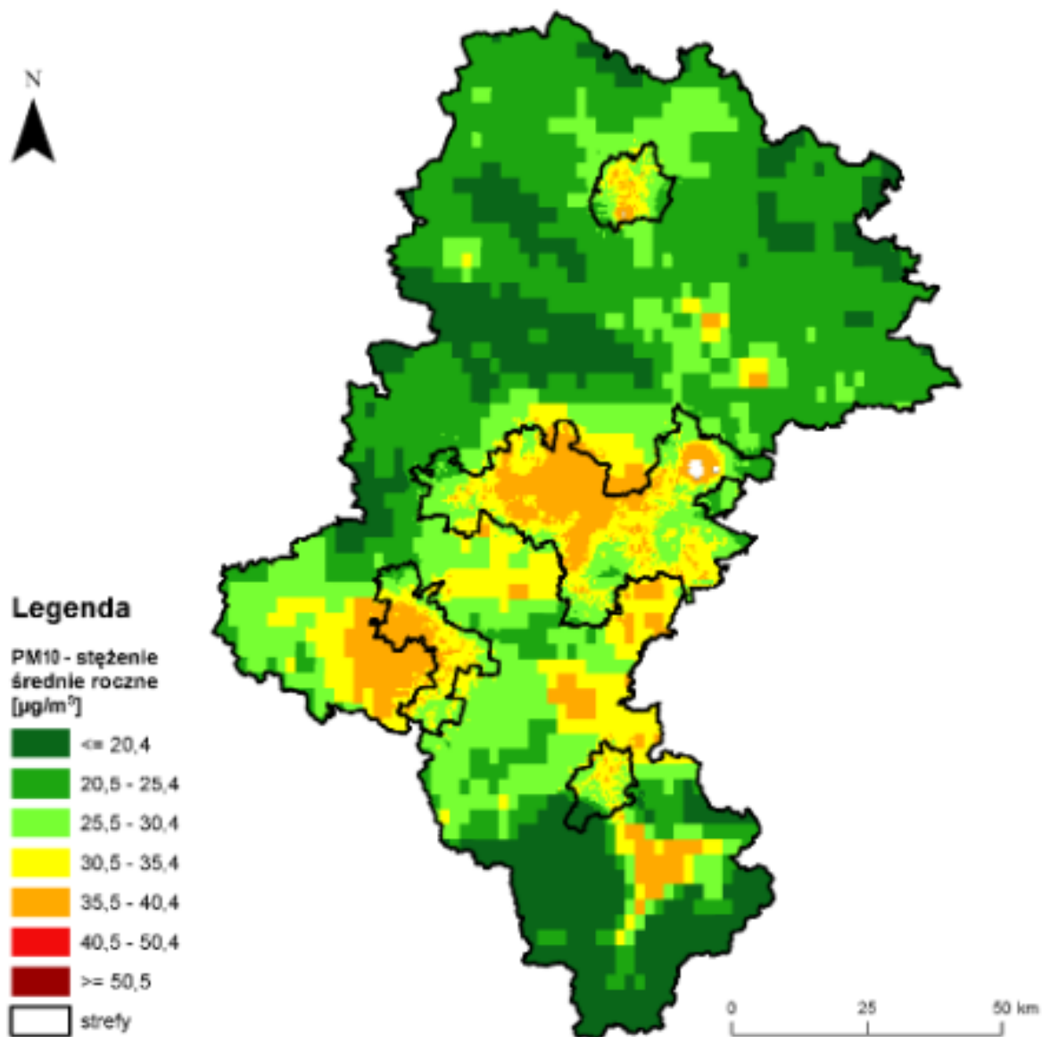
Mapa 23. Rozkład przestrzenny średniorocznego stężenia pyłu PM10 na obszarze województwa śląskiego w 2021 roku.
